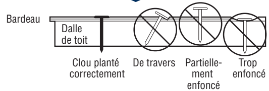
Figure 15-5 : Clouage adéquat et non adéquat
