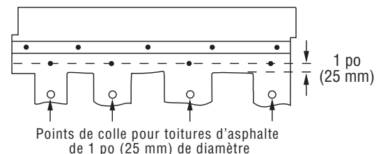
Figure 15-7 : Fixation des bardeaux Presidential et Presidential TL sur les pentes raides.
