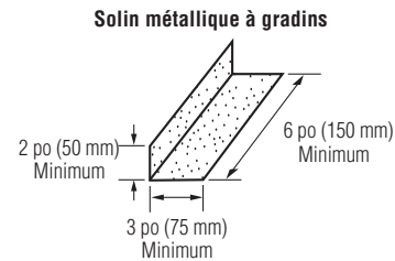
Figure 15-23 : Solin métallique à gradins.
