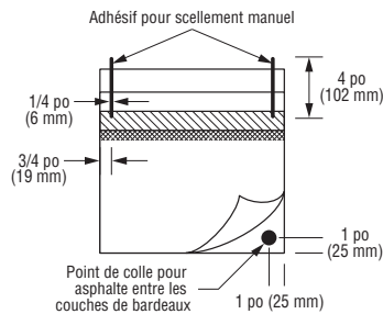
Figure 15-22 : Sceller les bardeaux de faîtage à la main de la façon indiquée.
