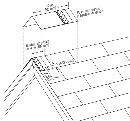
Figure 15-20 : Poser un bardeau de faîtage entier par-dessus le bardeau de départ.
