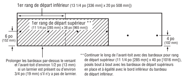
Figure 15-11 : Utiliser deux couches de pièces « Presidential Starter » de CertainTeed en chevauchement.
