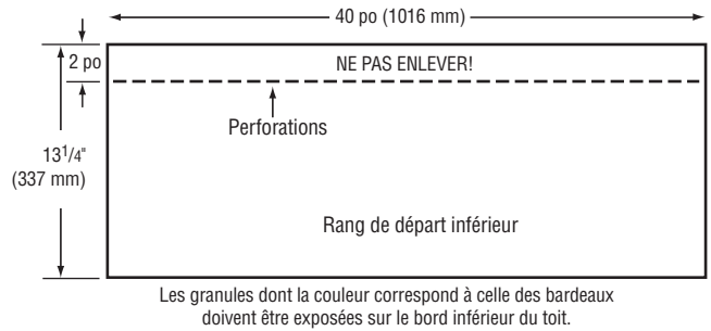
Figure 15-9 : Bardeau de départ Presidential (rang de départ inférieur).
