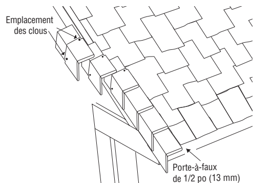
Figure 15-18 : Recouvrement des versants avec Mountain Ridge.
