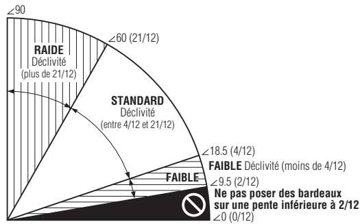
Figure 15-4 : Définition des pentes.
