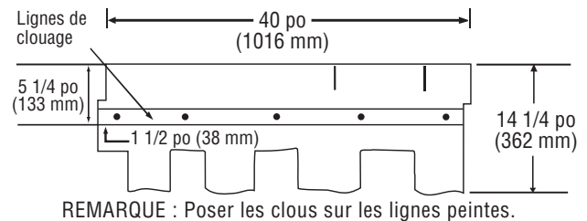
Figure 15-6 : Fixation des bardeaux Presidential et Presidential TL sur les pentes faibles et standards.
