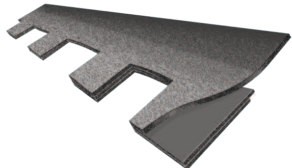
Figure 15-3 : Couches du Presidential TL.
