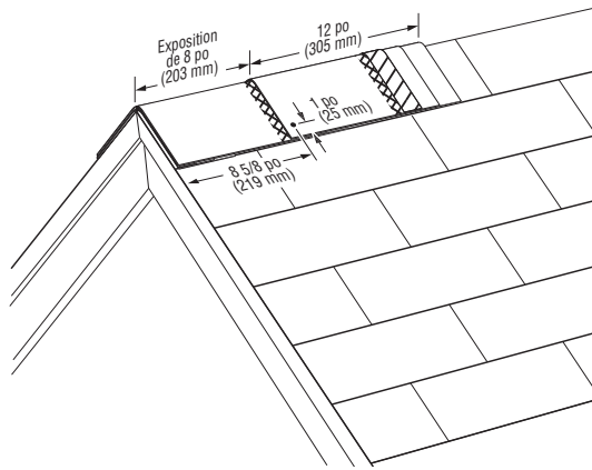
Figure 15-21 : Poser les bardeaux de faîtage en laissant une exposition de 8 po (203 mm) et planter un clou de chaque côté de la façon indiquée.
