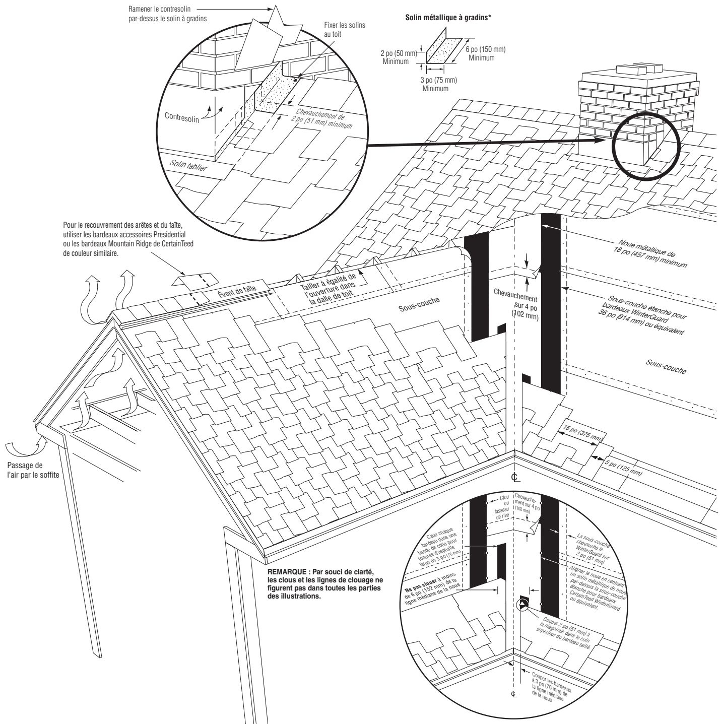
Figure 15-16 : Détail des solins de noue ouverte et de cheminée.
