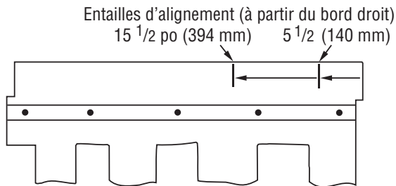
Figure 15-8 : Utiliser les entailles d'alignement pour assurer que les bardeaux sont posés à un décalage diagonal de 5 po (127 mm) et de 15 po (380 mm).
