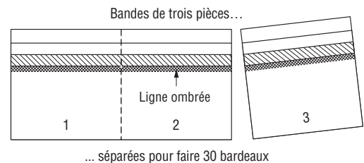
Figure 15-19 : Séparer pour obtenir trois bardeaux de faîtage.
