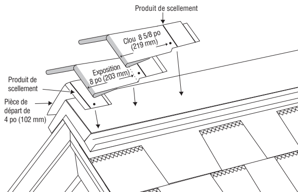
Figure 15-17 : Recouvrement d'arête et de faîte avec Mountain Ridge.
