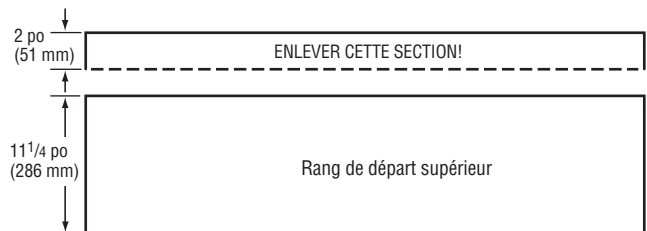
Figure 15-10 : Bardeau de départ Presidential (rang de départ supérieur).
