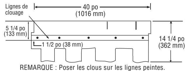
Figure 15-6 : Fixation des bardeaux Presidential et Presidential TL sur les pentes faibles et standards.
